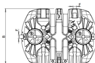
Vue de dessus de la FTE03000BI
