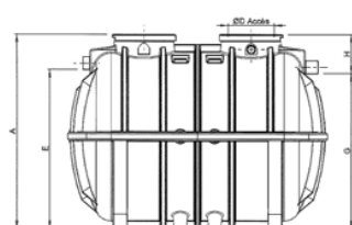
Vue latérale de la FTE2/6309/10
