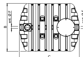
Vue de dessus de la INR06000 et INR08000
