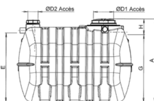
Vue latérale de la FTE2/6009/05 (pour BIONUT2/6054/10)
