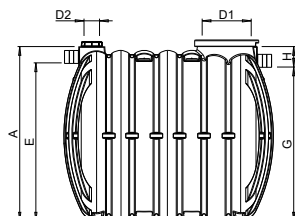
Vue latérale de la INR06000 et INR08000
