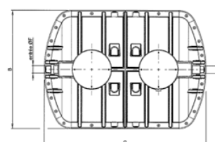
Vue de dessus de la FTE2/6309/10
